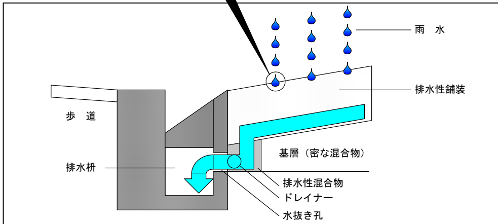
排水構造図
