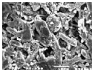
火山灰シラス壁 2,000倍顕微鏡写真
